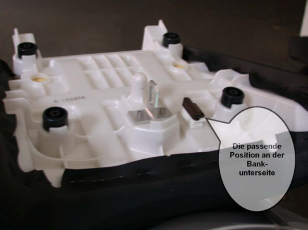
Bild 8: Passend zu dem am Fahrzeug montierten Kontakt das Gegenstück an der Sitzbank.
